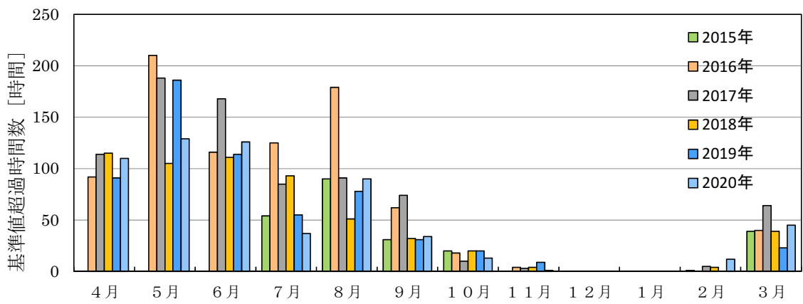
図 25 光化学オキシダントの基準値超過時間数
