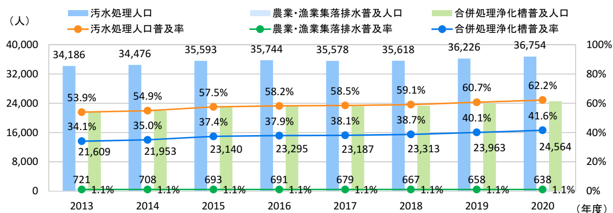
図 38 生活排水処理施設の普及状況の推移
