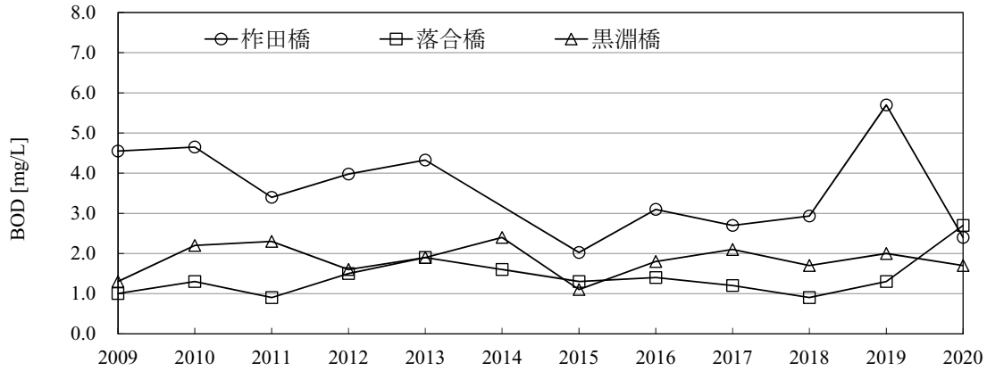
図 33 柞田川における BOD 年平均値の推移
