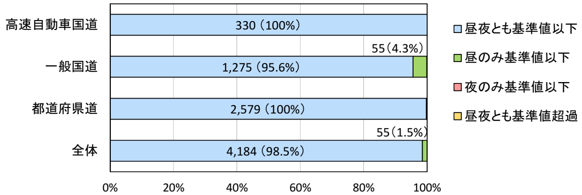
図 40 面的評価結果 (全体) (2012 年～2020 年実施分)
