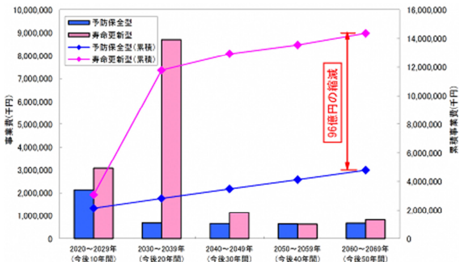
図 6.1 長寿命化修繕計画の効果
